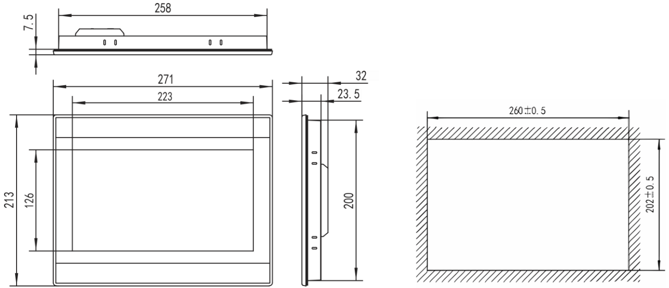
外形尺寸
