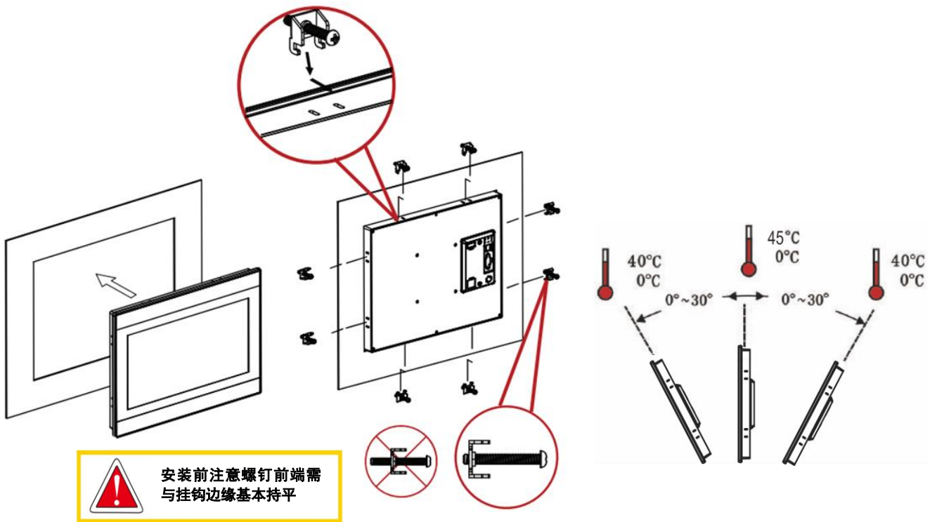
挂钩安装
